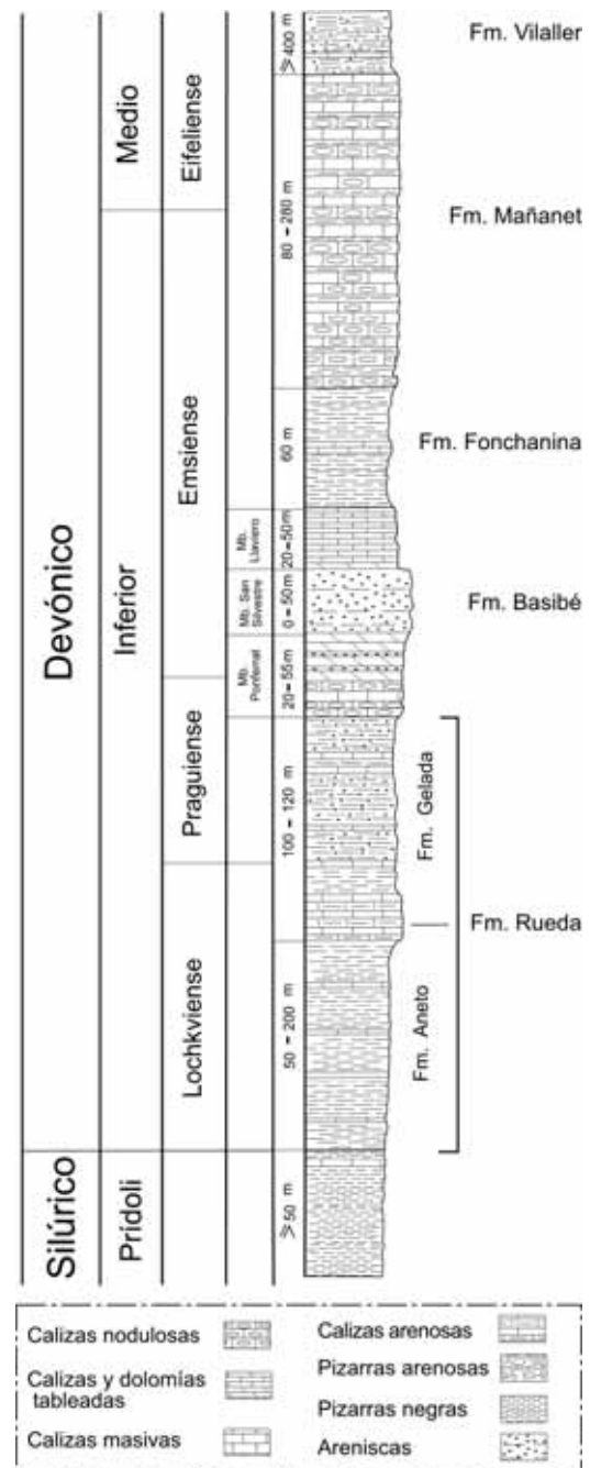
Figura 2. Columna sintética mostrando la estratigrafía de la facies Baliera (basado en Mey, 1967).
