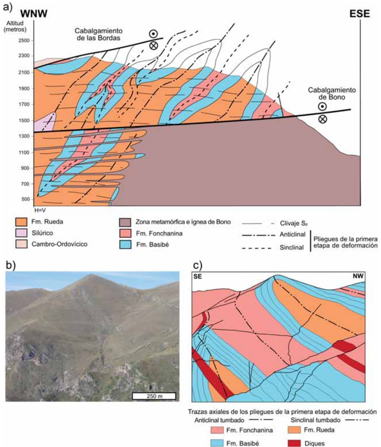
Figura 7. a) Corte geológico a través de la lámina cabalgante de Bono mostrando la disposición de los pliegues de la primera etapa de deformación y su replegamiento durante la segunda etapa de deformación; b) panorámica de la ladera NE del Pico del Mitch del Vedat; c) interpretación geológica de la panorámica donde se aprecian algunas de las características de los pliegues desarrollados durante la primera etapa de deformación.
