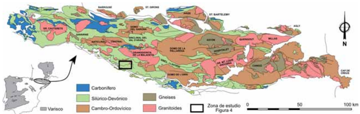
Figura 1. Esquema general de situación y mapa geológico simplificado de la Zona Axial Pirenaica (basado en García-Sanseguno, 1996). El recuadro corresponde al mapa de la figura 4.
