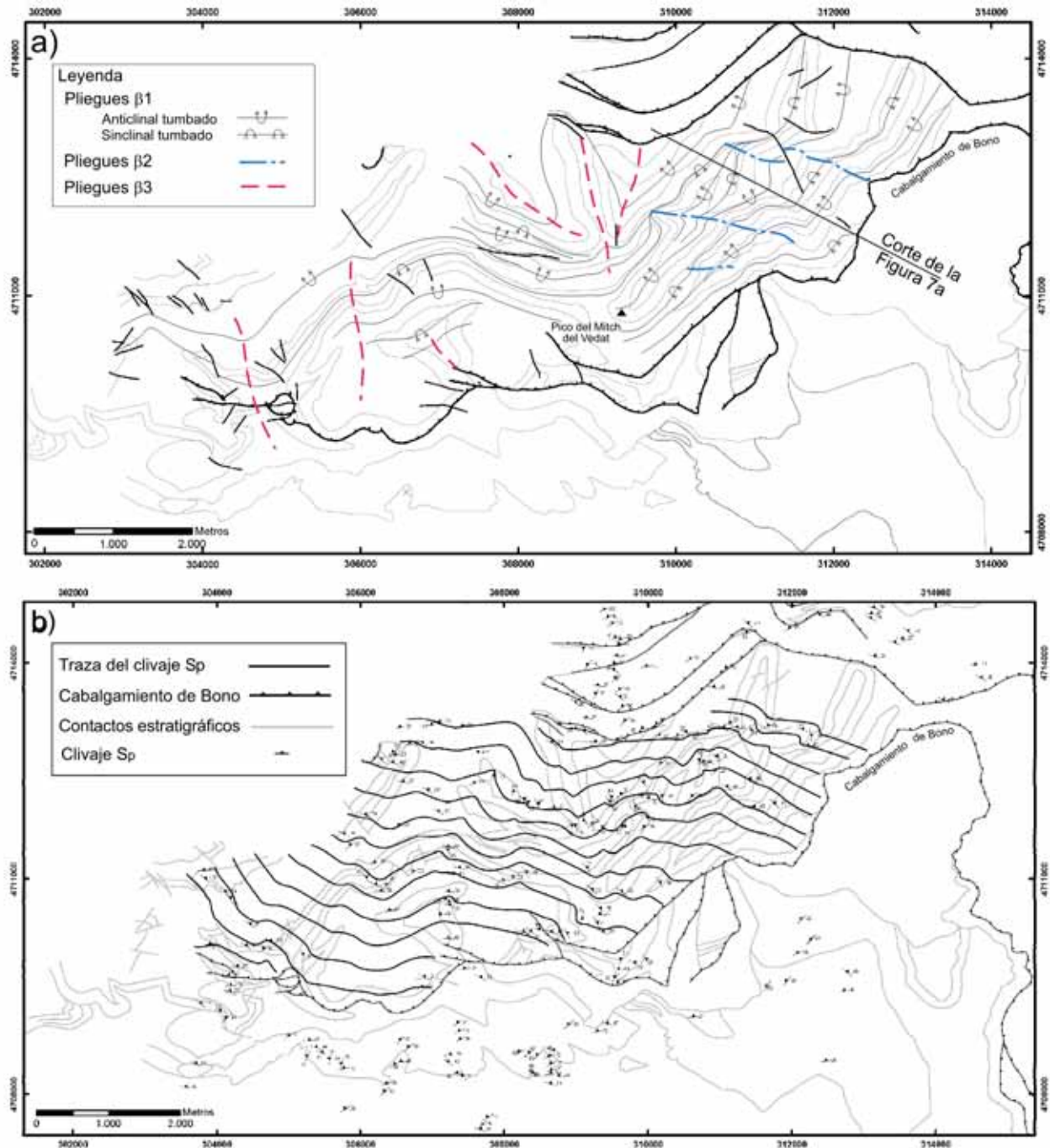
Figura 5. a) Esquema en el que se muestran las trazas axiales de los diferentes sistemas de pliegues: b1 (pliegues pertenecientes a la primera etapa de deformación), b2 (pliegues pertenecientes a la segunda etapa de deformación) y b3 (pliegues pertenecientes a la tercera etapa de deformación); b) Esquema de trazas del clivaje dominante ( S_p ) donde se aprecia claramente su oblicuidad con respecto a los pliegues b1 (de trazas axiales NE-SO).
