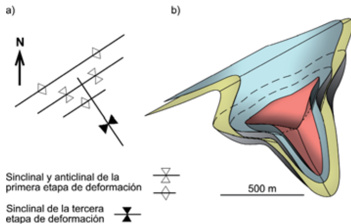
Figura 14. a) Esquema estructural de la superposición de pliegues de la primera etapa de deformación, con orientación NE-SO, y el sinformal tardío con orientación NNO-SSE en la zona del río Baliera; b) Reconstrucción tridimensional de dicha cubeta. Escala aproximada.
