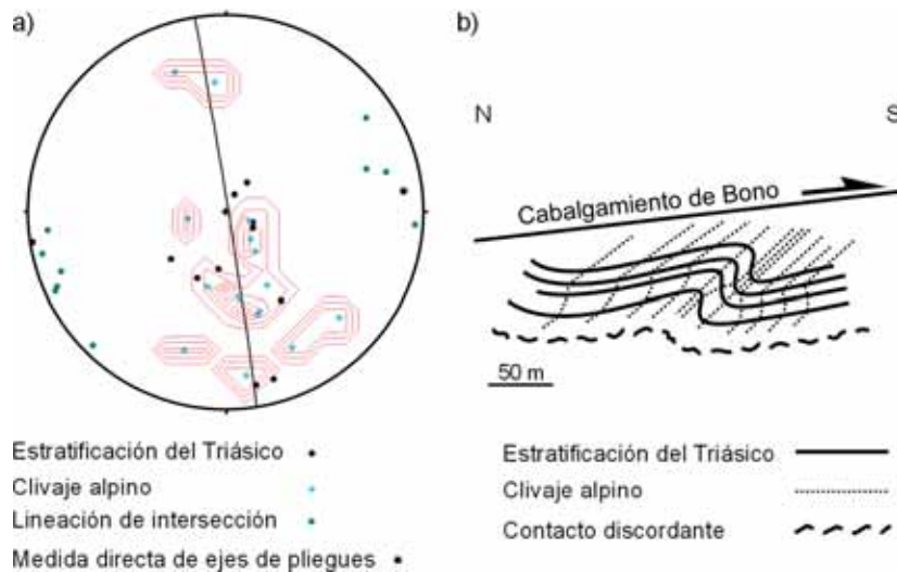
Figura 16. a) Proyección estereográfica con los datos de estratificación, clivaje alpino y lineación de intersección de los materiales triásicos; b) Esquema de los pliegues asimétricos y el clivaje asociado a ellos en los materiales triásicos que se encuentran en el bloque de muro del cabalgamiento de Bono.
