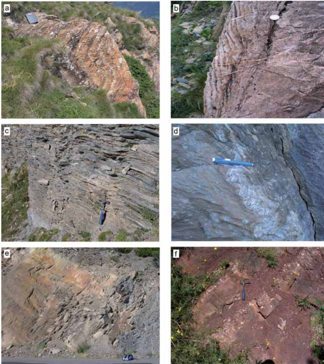
Figura 3. Aspecto de campo de las diferentes formaciones presentes en la zona de estudio. a) Calizas basales de la Formación Basibé en las que se observa un pequeño pliegue con un clivaje de plano axial asociado; b) miembro cuarácítico de la Formación Basibé el cual presenta una estratificación cruzada; c) calizas negras tableadas del miembro superior de la Formación Basibé; d) calizas de la Formación Mañanet donde se aprecia como el clivaje (paralelo al lápiz azul), deforma los planos de estratificación; e) pizarras de la Formación Vilaller con la estratificación inclinada hacia la derecha de la fotografía y el clivaje inclinado hacia la izquierda de la misma; f) conglomerados y areniscas del Triásico inferior en facies Buntsandstein donde se aprecia un ligero clivaje hacia la derecha de la fotografía.
