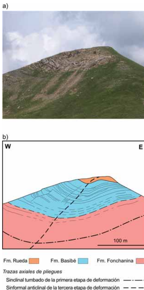
Figura 13. a) Vista al norte del sinformal-anticlinal en cuyo núcleo aflora la Formación Rueda y en sus flancos la Formación Basibé y la Formación Fonchanina; b) Interpretación geológica de la fotografía. Escala aproximada.
